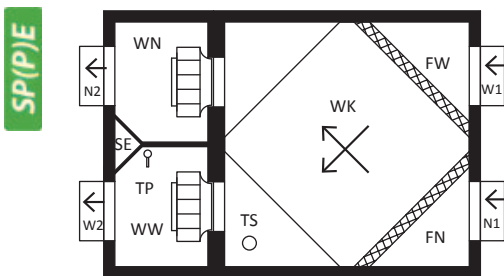
widok z góry / wykonanie centrali „prawe” (MMK-SP(P)E)
