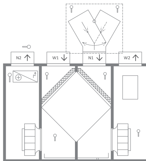
widok z przodu / wykonanie centrali „lewe” (RK-UPEL)
