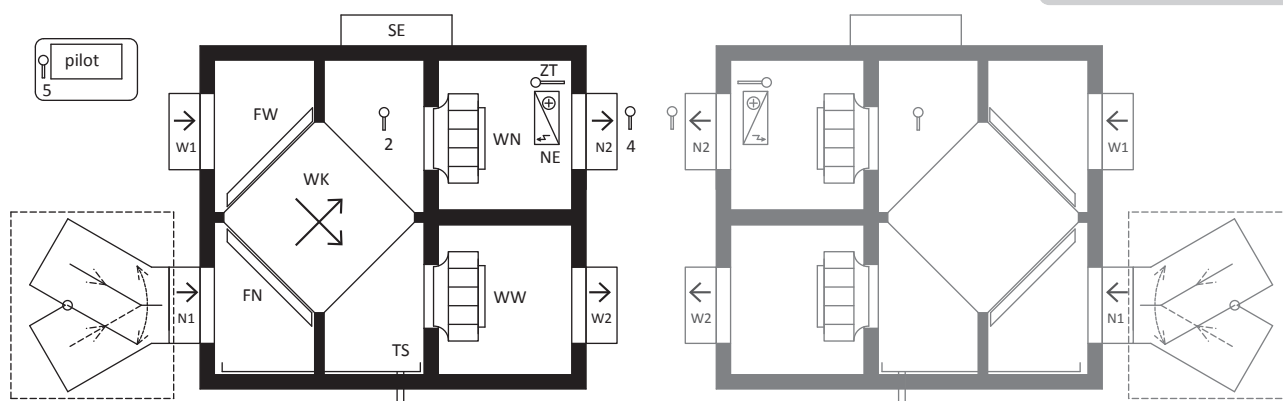
widok z przodu / wykonanie centrali „prawe” (RK-KP)
