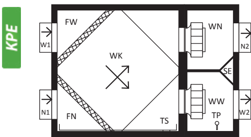
widok z przodu / wykonanie centrali „prawe” (MMK-KPE)
